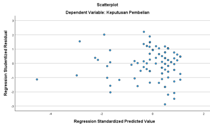
Gambar 3. Uji Heteroskedastisitas
