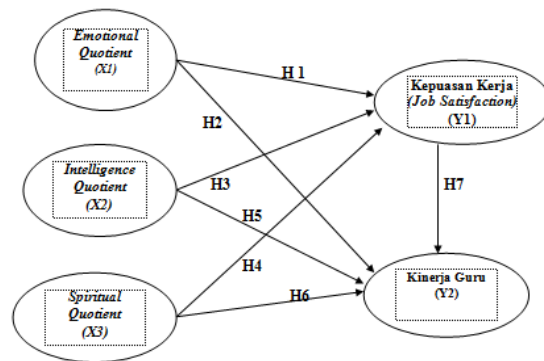
Gambar 1. kerangka pikir
